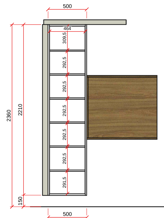
VISTA D - ESC. 1:30
