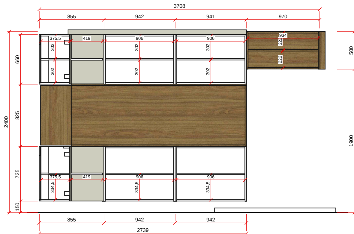
VISTA C - ESC. 1:30
