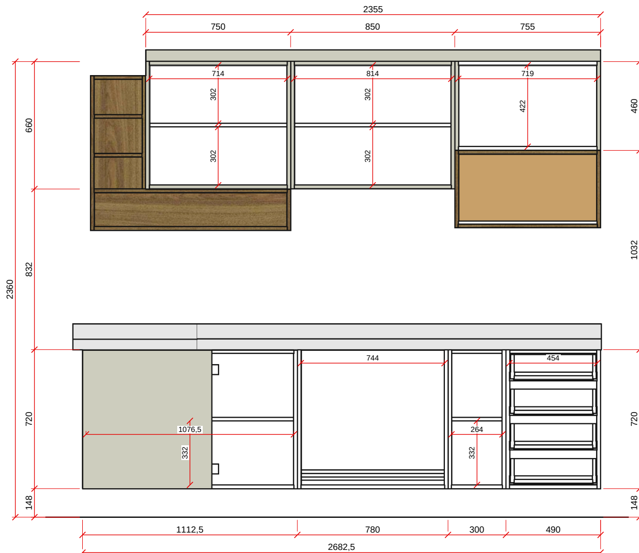
VISTA A - ESC. 1:20
