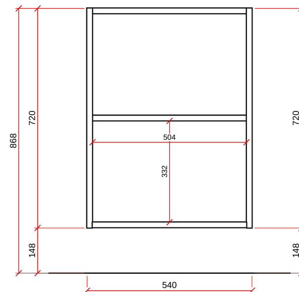
VISTA B - ESC. 1:12.5
